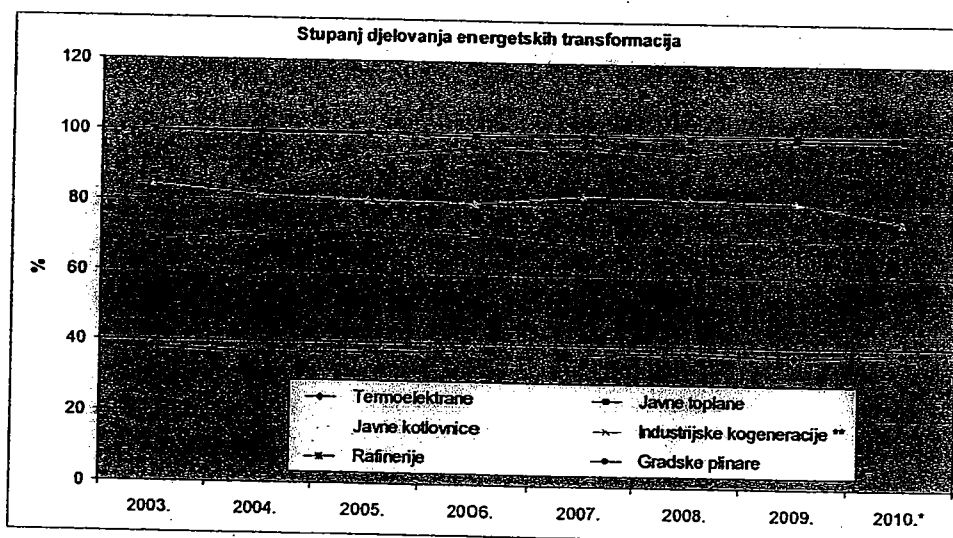
Slika 9. Učinkovitost energetske transformacije
